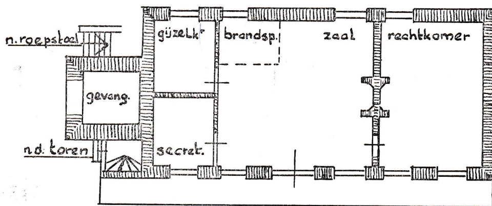
begane grond voor de verbouwing van 1786
