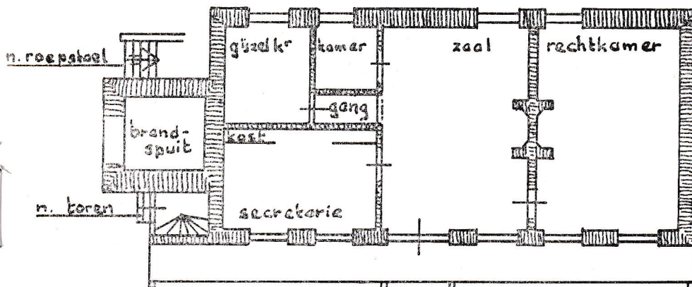
begane grond na de verbouwing van 1786/1787
